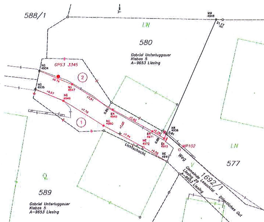
Abb. 1: Ausschnitt aus der Vermessungsurkunde betreffend Aufhebung der Widmung zum Gemeindegebrauch; Abbildung nicht maßstabsgetreu!
