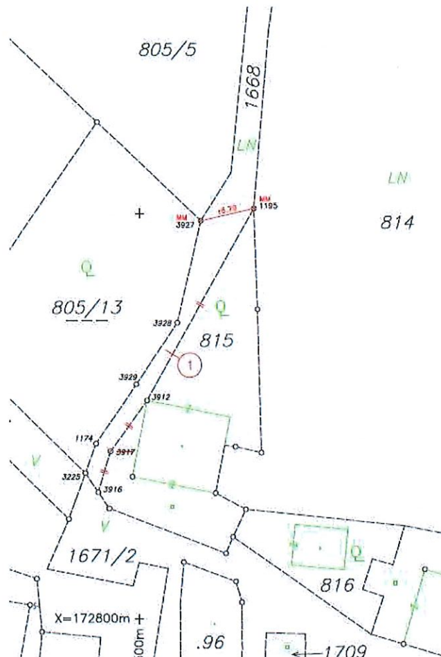
Abbildung 1: Ausschnitt aus der Vermessungsurkunde betreffend Aufhebung der Widmung zum Gemeindegebrauch; Abbildung nicht maßstabsgetreu!
